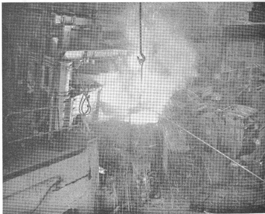
Ståltappning vid ljusbågeugn i SKF Katrineholmsverken.
